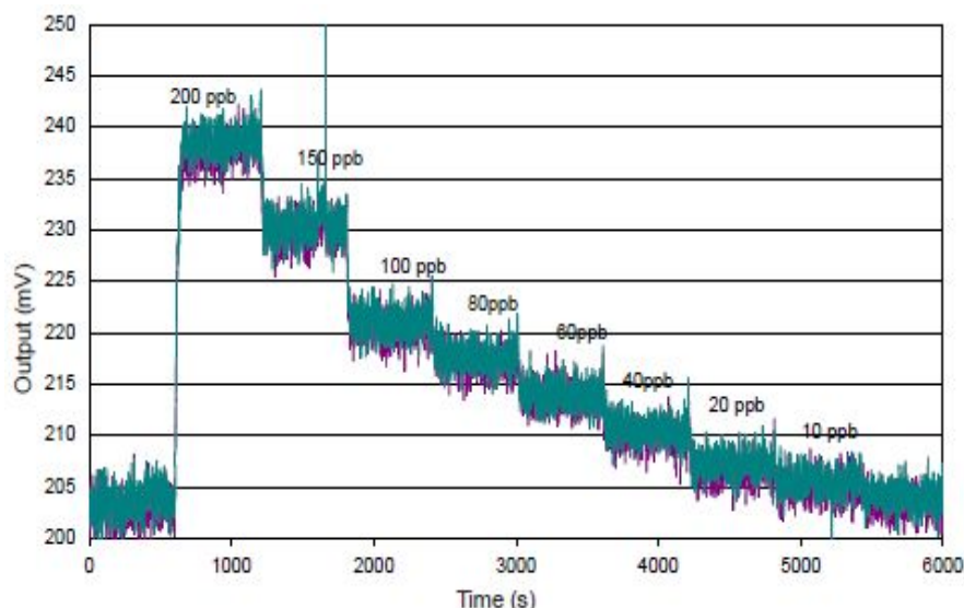
图4 对200ppb NO 2 的反应
