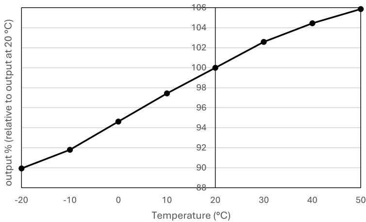
图2 灵敏度温度特性
