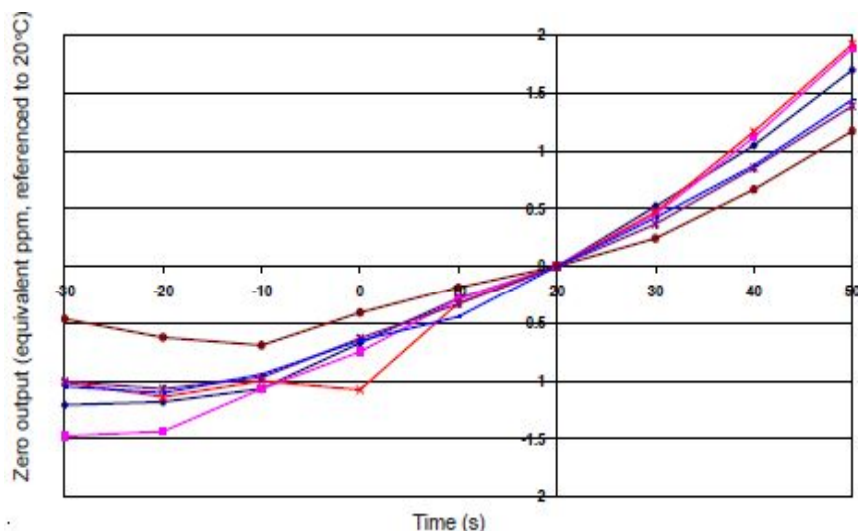
图4 批量传感器输出的可重复性
