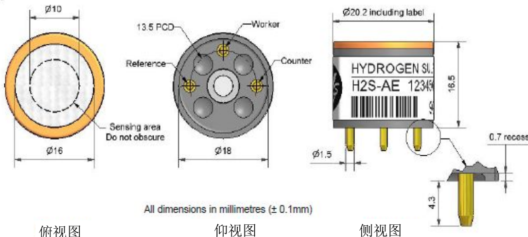
图1 H2S-AE示意图
