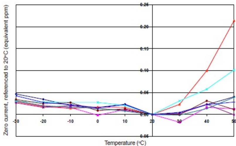
图6 H 2 S通道零点温度特性
