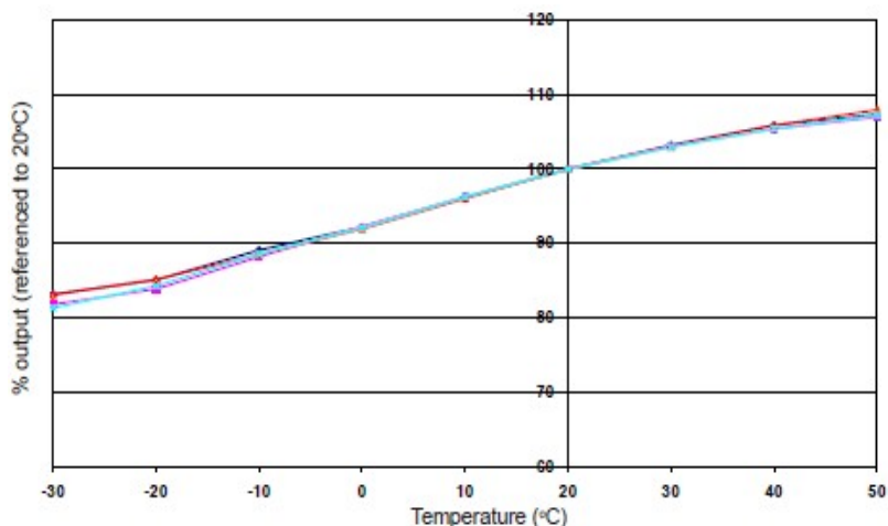
图5 H 2 S通道灵敏度温度特性
