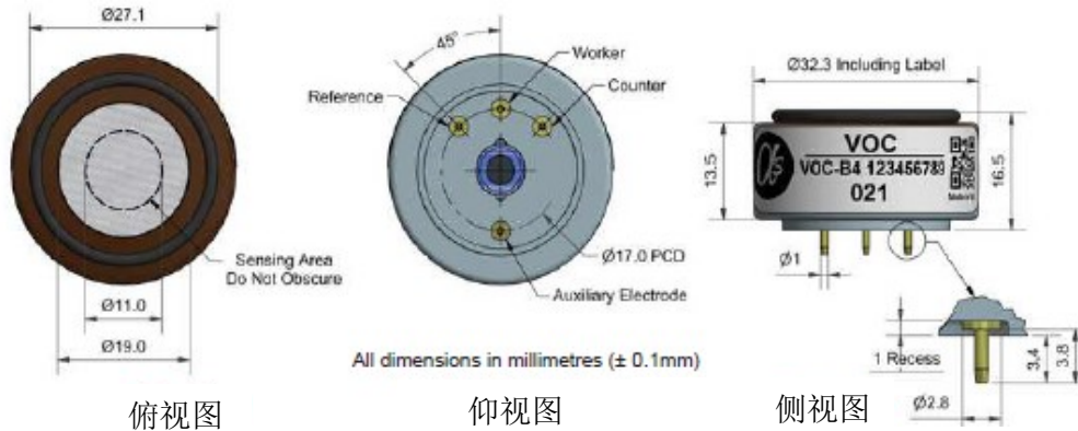
图1 VOC-B4示意图
