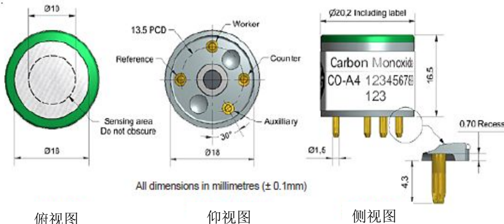
图1 CO-A4示意图
