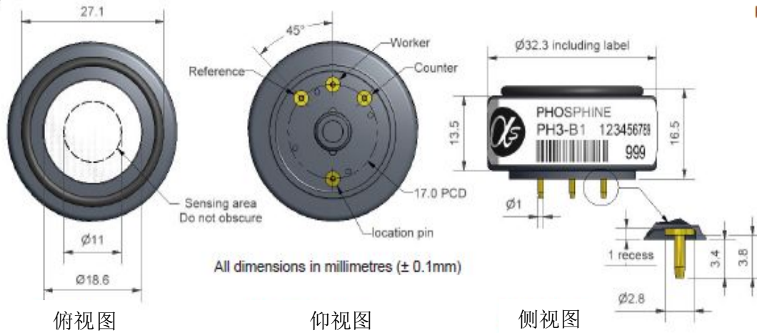
图1 PH3-B1示意图
