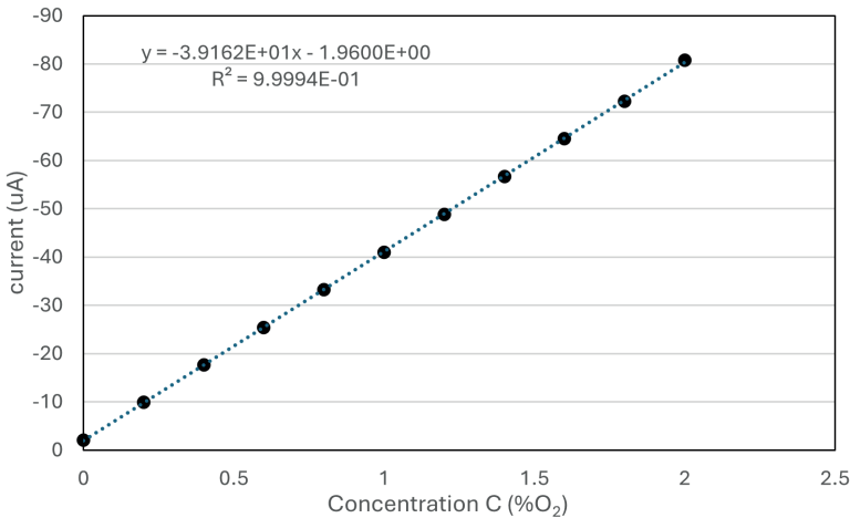
图3 线性度(0 - 2% 氧气)
