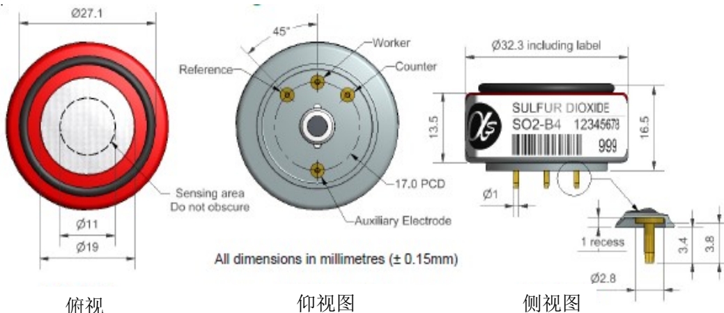
图1 SO2-B4示意图
