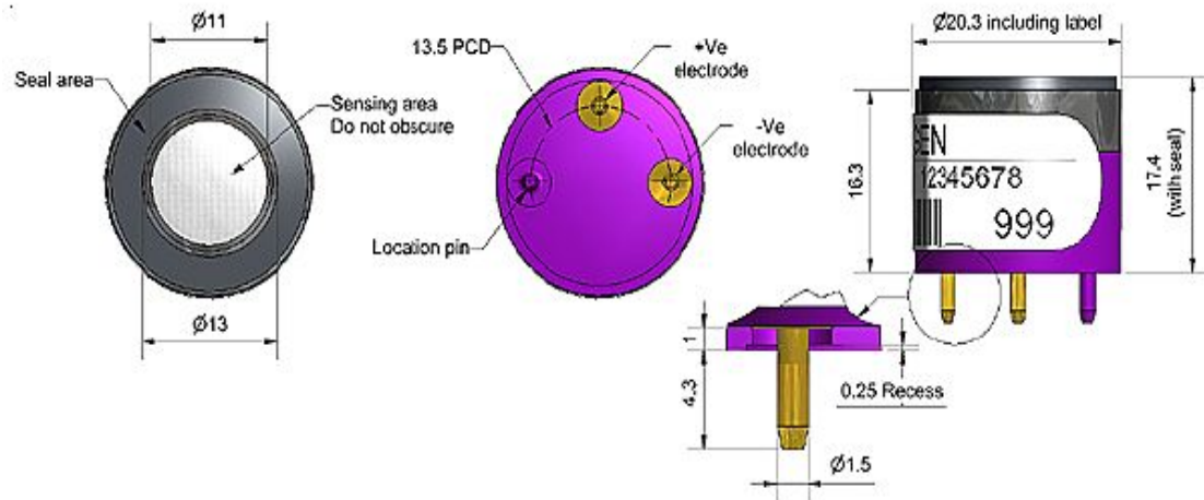
图1 O2-M2 示意图
