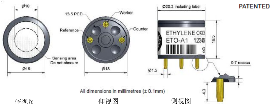
图1 ETO-A1 示意图
