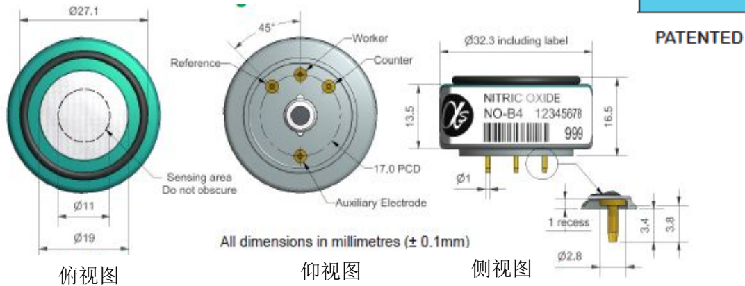
图1 NO-B4示意图
