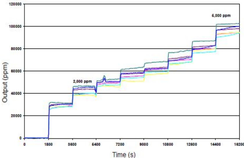
图4 过载线性度
