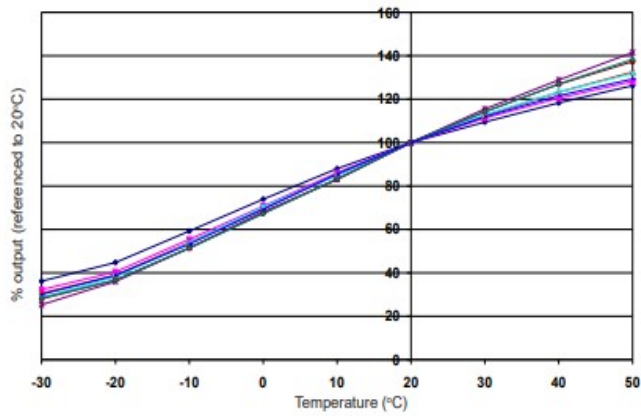
图1 CO通道灵敏度温度特性
