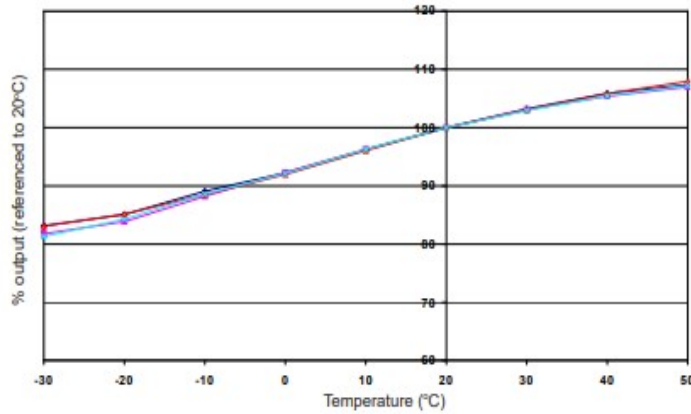
图5 H 2 S通道灵敏度温度特性
