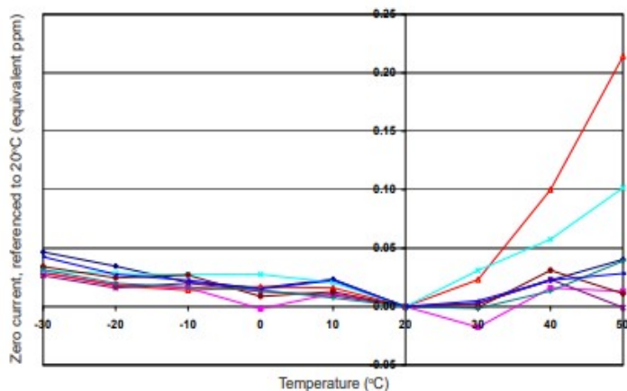
图6 H 2 S通道零点温度特性
