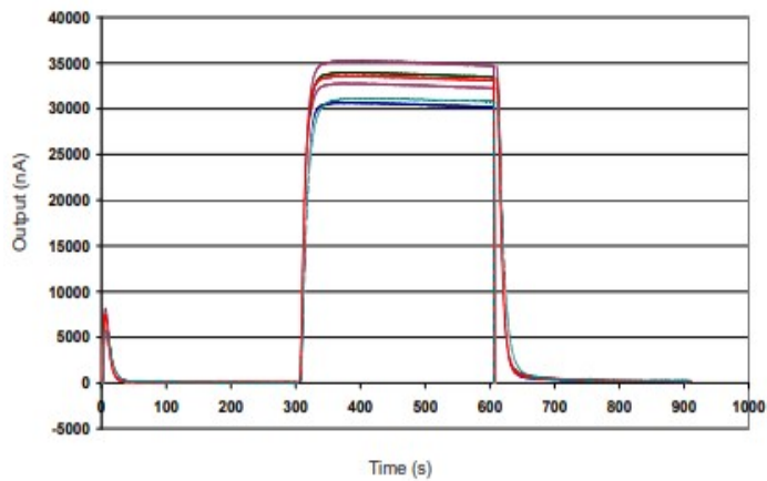
图3 CO通道对400ppm CO的反应
