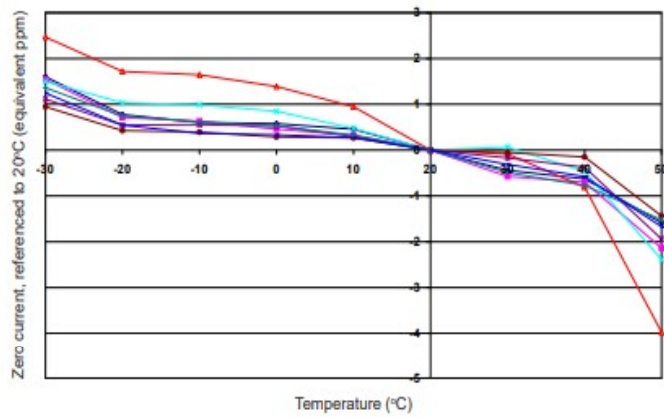
图2 CO通道零点温度特性
