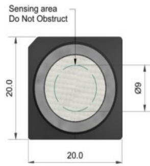
顶视图
