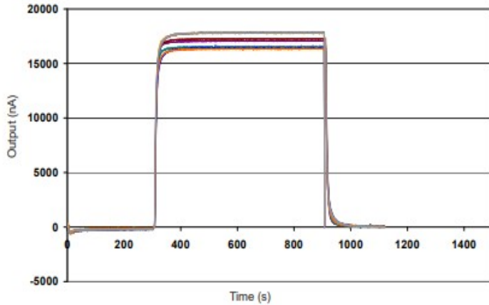
图4 H 2 S通道对25ppm H 2 S的反应
