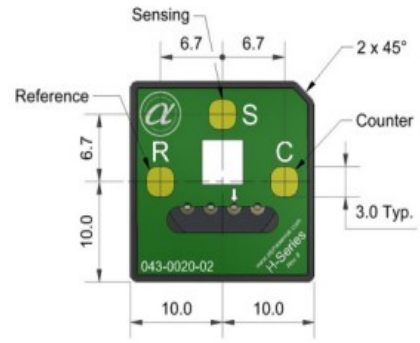
底视图
