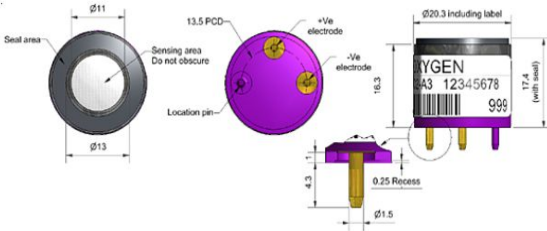
图1 O2-A3示意图
