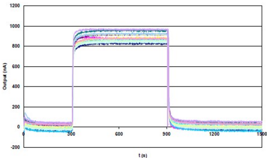
图3 对 25ppm HCN 的反应
