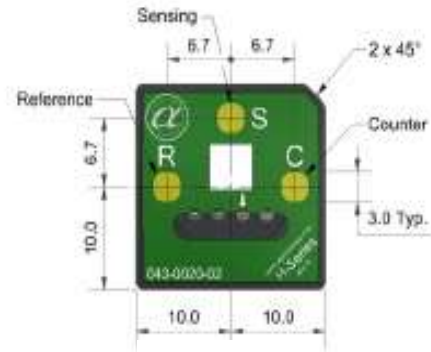
底视图
